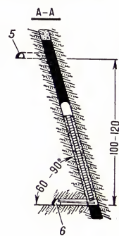
Рис. 15. Система разработки горизонтальными полосами по простиранию в восходящем порядке: 1 — конвейерный квершлаг; 2 — вентиляционный скат; 3 — вентиляционный квершлаг; 4 — углеспускной скат; 5 — слоевой вентиляционный штрек; 6 — слоевой откаточный штрек.
